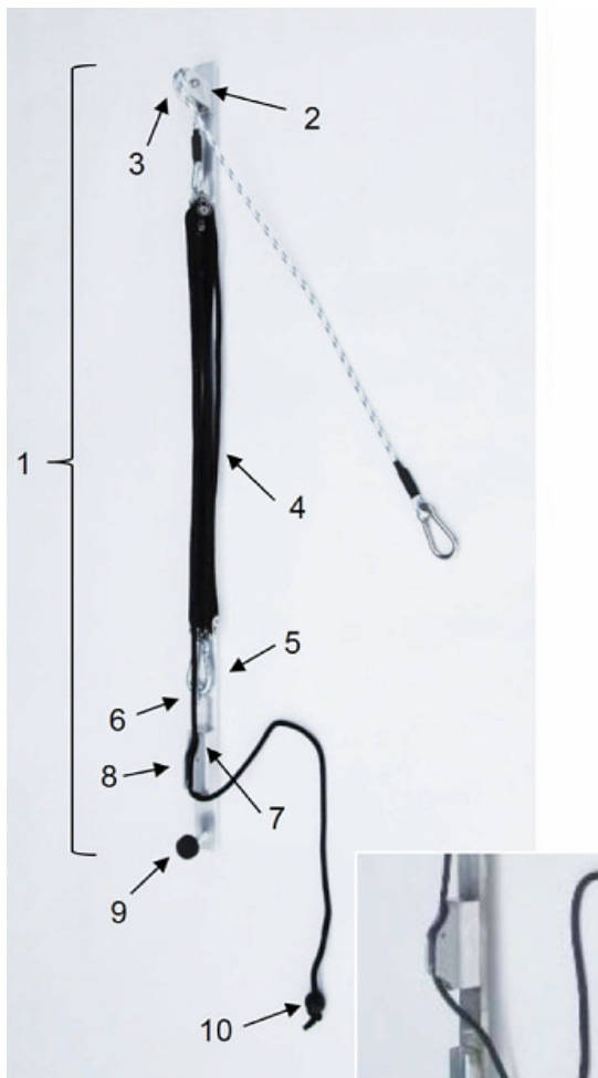
Mechanikschieber
