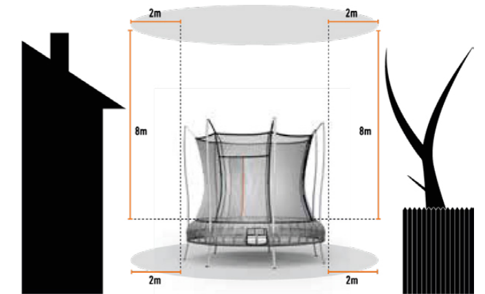
INSTALLAZIONE CORRETTA
